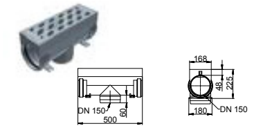
Vertikalt utlopp
