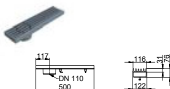
Utloppselement
