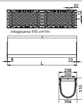
Baselement
