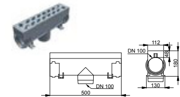
Vertikalt utlopp
