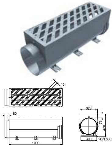
Baselement
