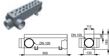
Sidoutlopp front / vänster / höger
