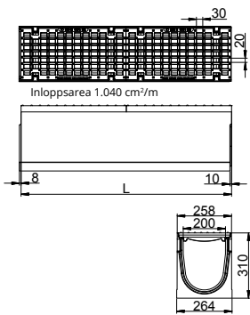
Baselement
