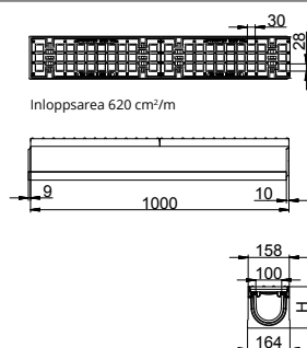
Baselement
