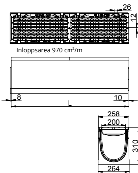
Baselement
