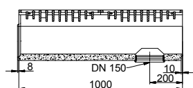
Utloppselement
