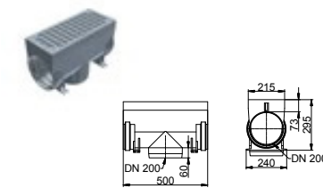
Vertikalt utlopp
