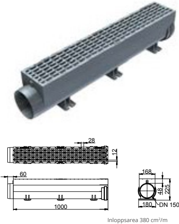
Baselement
