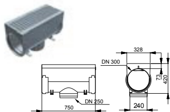
Vertikalt utlopp
