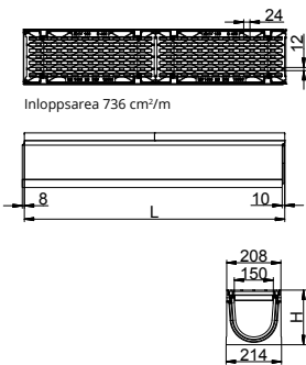
Baselement
