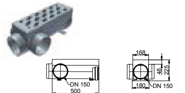
Sidoutlopp front / vänster / höger
