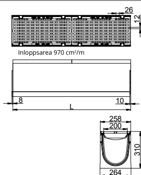
Baselement
