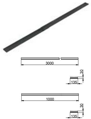
Baselement
