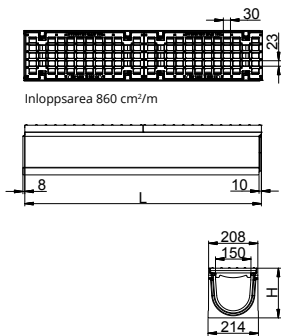
Baselement
