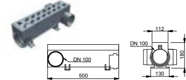
Sidoutlopp vänster /höger
