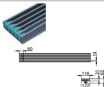
Rengöringselement
