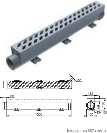
Baselement
