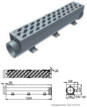
Baselement
