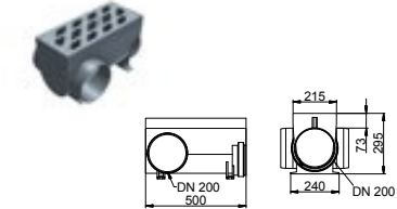
Sidoutlopp vänster /höger
