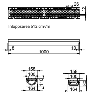
Baselement
