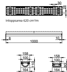
Baselement
