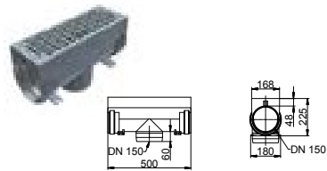
Vertikalt utlopp
